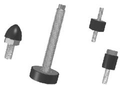
Gummistopfen nach Kundenzeichnung
